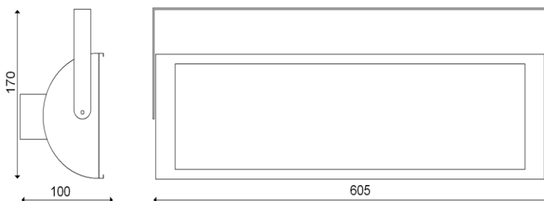
Encombremments
